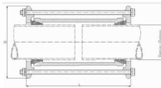
rys.2 korpus łącznika żeliwo
