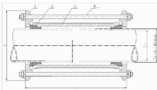
rys.1 korpus łącznika PE- HD NOWOŚĆ
